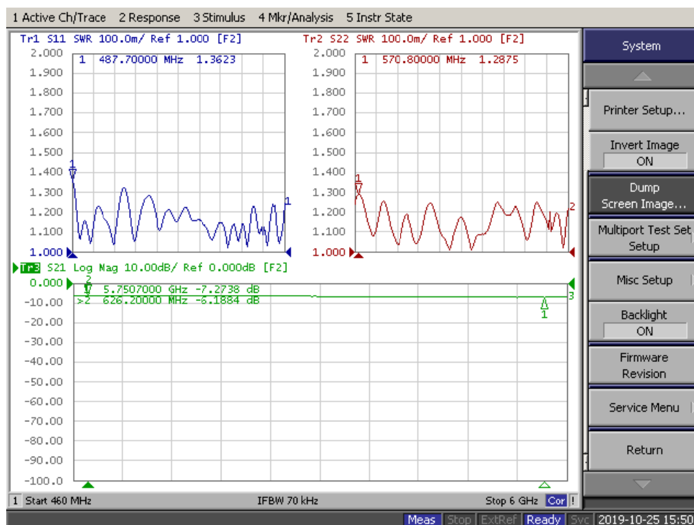
TR1: SUM Port VSWR, TR2: P4 Port VSWR, TR3: SUM-P4 Port Insertion Loss
