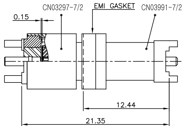
체결도 (SCALE 3:1)
