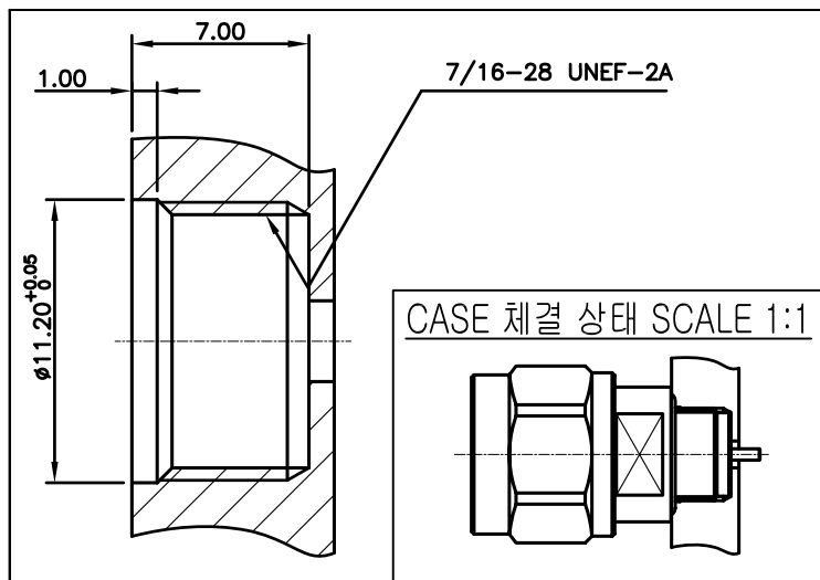
CASE 체결 치수
