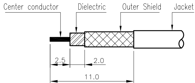
CABLE 탈피도
