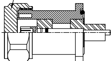
CN00785-7/1 도장용 DUST CAP
