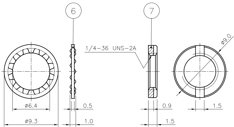
WASHER 별도 포장 (SCALE 3/1)
