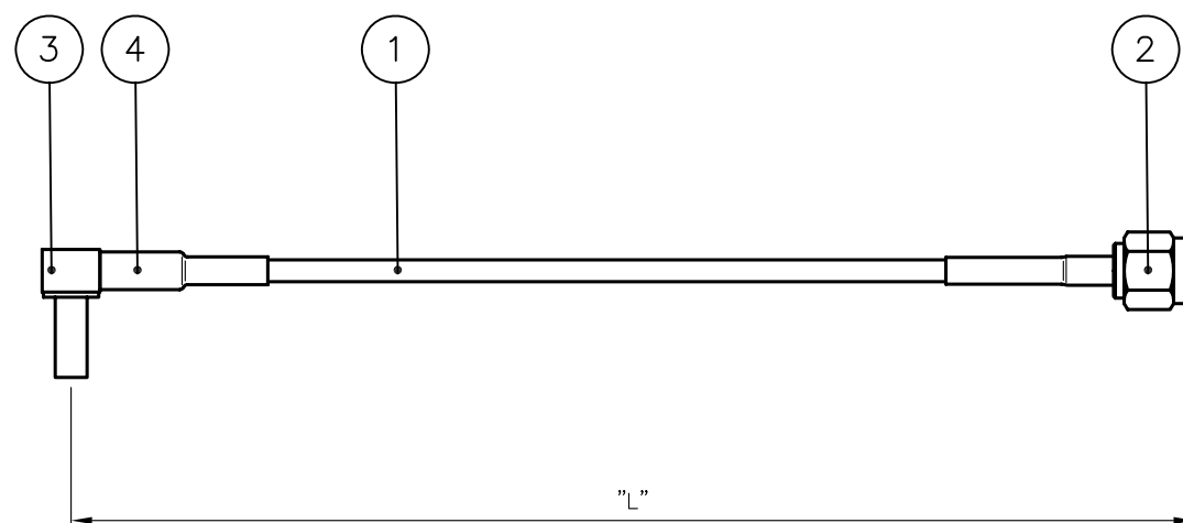
2번 Conn CABLE 탈피도
