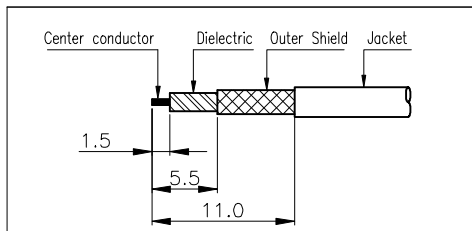
②번 CABLE 탈피도
