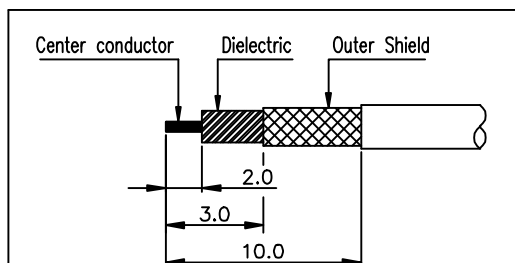
2번 CONNECTOR 탈피도
