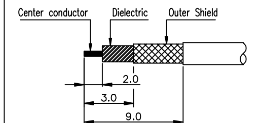
3번 CONNECTOR 탈피도
