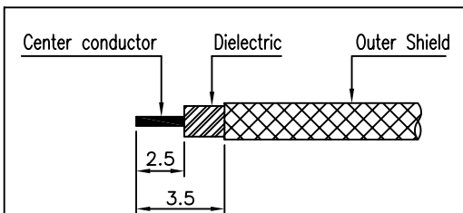
② Connector 탈피도
