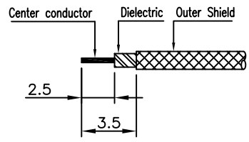
③ CABLE 탈피도
