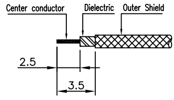
② CABLE 탈피도
