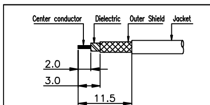
③번 CONNECTOR 활피도
