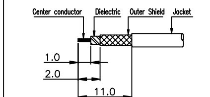
②번 CONNECTOR 활피도
