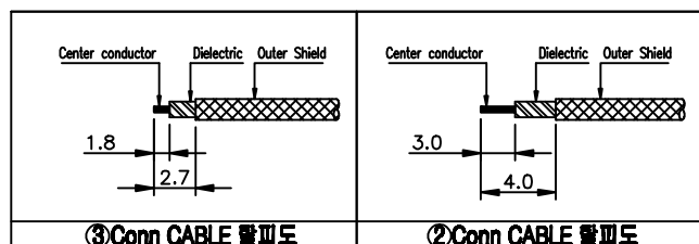
③Conn CABLE 할피도
