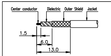
③번 CABLE 할피도
