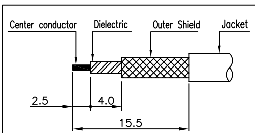
③ CABLE 탈피도
