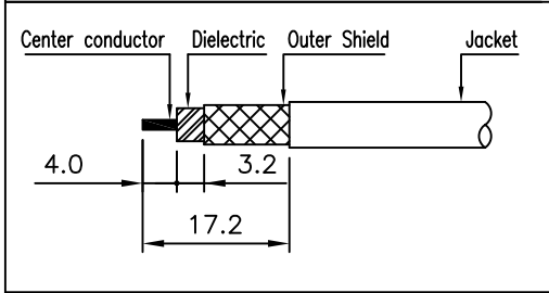
② CABLE 탈피도
