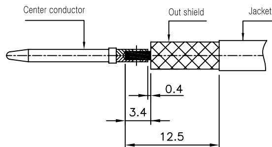
2번 CONNECTOR 탈피도
