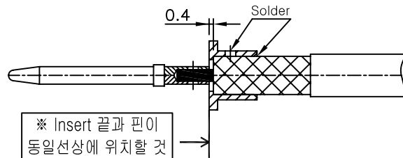
N Type 케이블 심선+핀 조립
