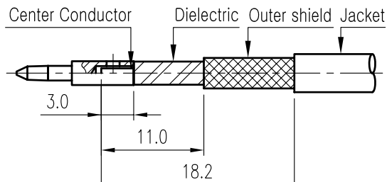
2번 Conn CABLE 탈피도
