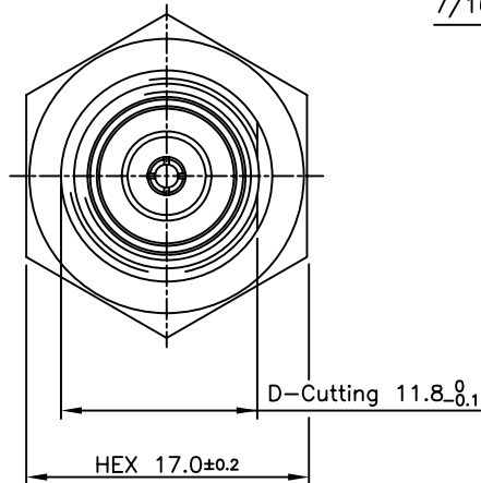
CABLE 탈피도
