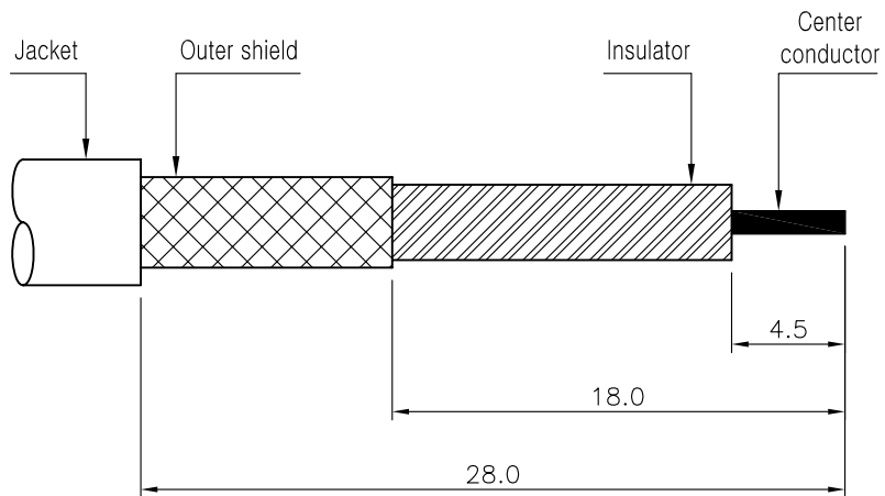
CABLE 탈피도
