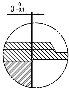
A부 확대도
