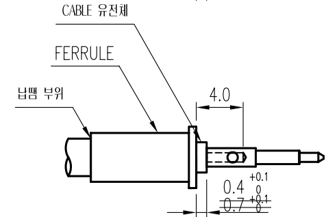
2. CABLE ASS'Y도
