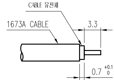
1. CABLE ASS'Y 탈피도
