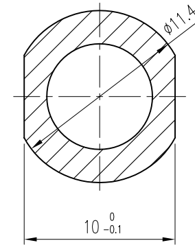
단 면 A - A
