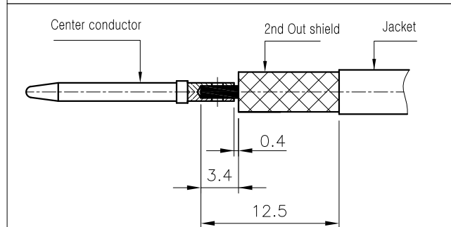
2번 CONNECTOR 탈피도
