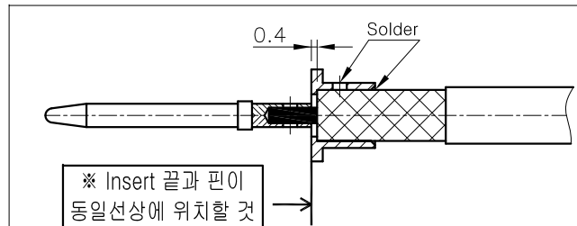
N Type 케이블 심선+핀 조립
