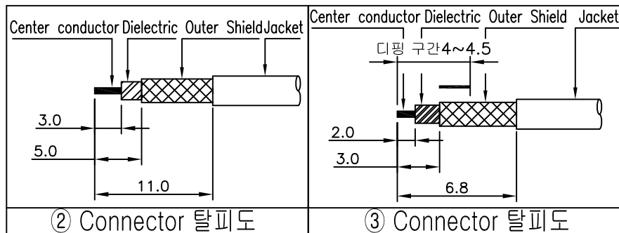
QMA 압착 사이즈
