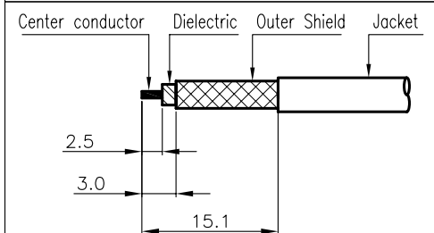
3번 Conn CABLE 탈피도
