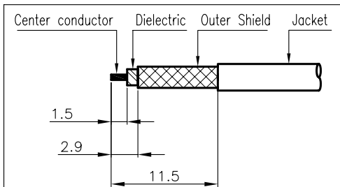
2번 Conn CABLE 탈피도
