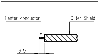
No.2 Conn CABLE 탈피도
