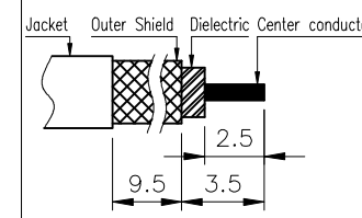
3번 Conn CABLE 탈피도
