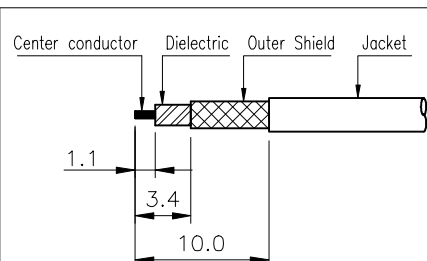
③번 Connector 탈피도
