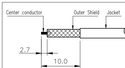
②번 Connector 탈피도
