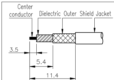
2번 CONNECTOR 탈피도
