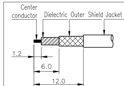
3번 CONNECTOR 탈피도
