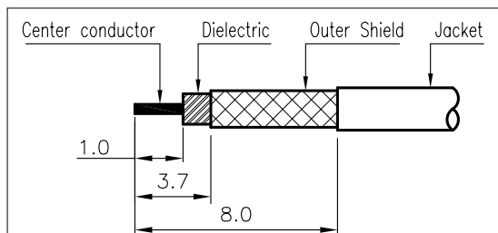
③번 CONNECTOR 탈피도
