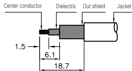
3번 CONNECTOR 탈피도
