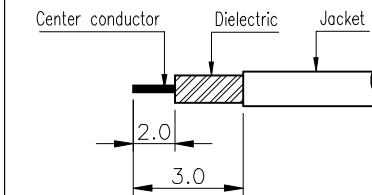
③번 CONNECTOR 탈피도
