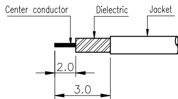
②번 CONNECTOR 탈피도
