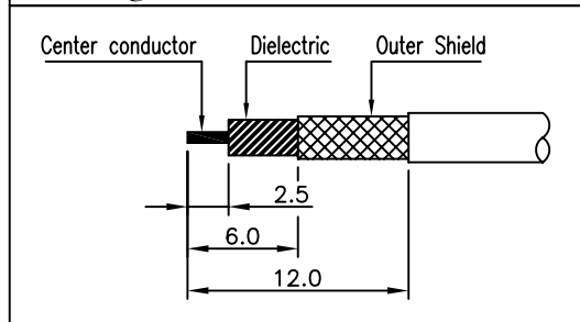
③ Conn CABLE 탈피도
