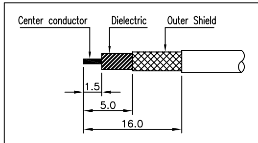
② Conn CABLE 탈피도
