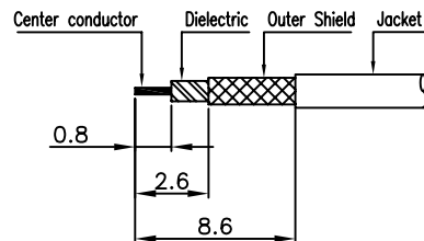
③번 Conn CABLE 탈피도
