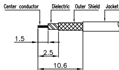
②번 CABLE 탈피도
