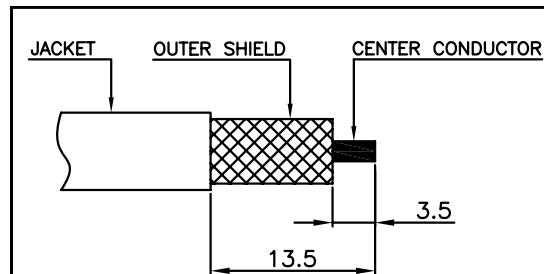
② Conn CABLE 탈피도
