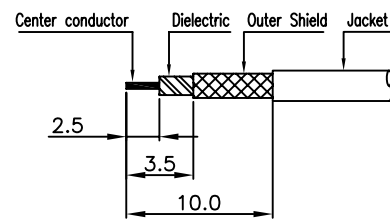
②번 CABLE 탈피도
