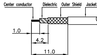
③번 CABLE 탈피도
