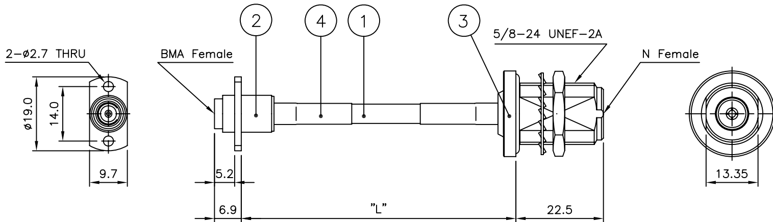
2번 Conn CABLE 탈피도
