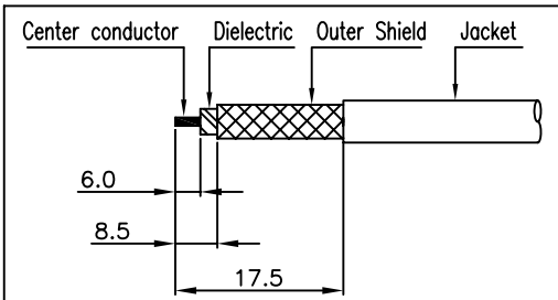
② Connector 탈피도
