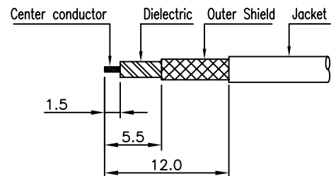
③ CONNECTOR 탈피도
