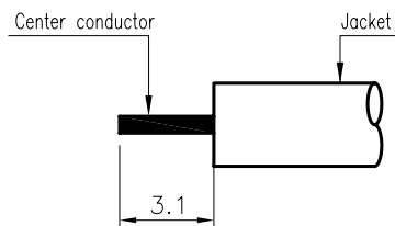
3번 Conn CABLE 탈피도
