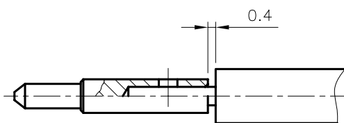
2번 Conn CABLE 탈피도
