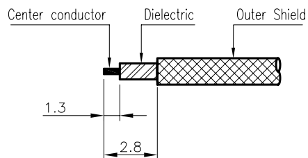
2번 Conn CABLE 탈피도
