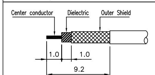
③번 CABLE 탈피도
