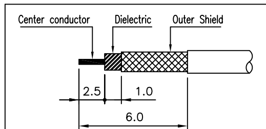
②번 CABLE 탈피도
