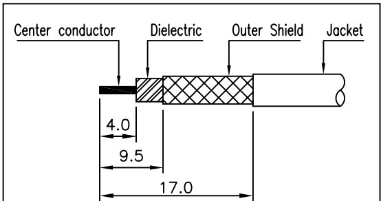
② Conn CABLE 탈피도
