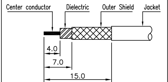
③ Conn CABLE 탈피도
