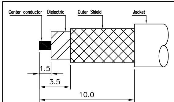
②번 CONNECTOR 탈피도
