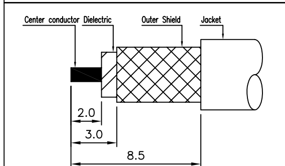
③번 CONNECTOR 탈피도
