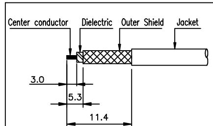
2번 Conn CABLE 탈피도
