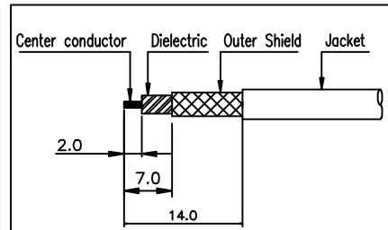
3번 Conn CABLE 탈피도
