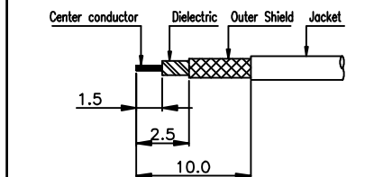
②번 CABLE 발피도
