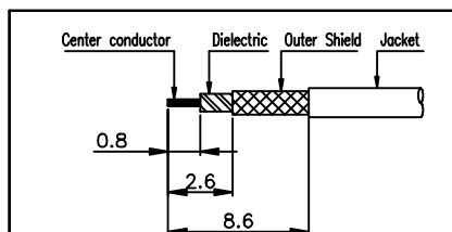
③번 Conn CABLE 탈피도
