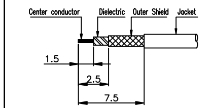
②번 CABLE 탈피도
