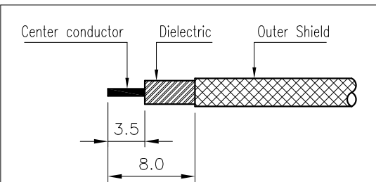
③번 CONNECTOR 탈피도
