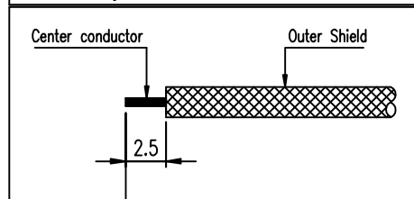
②번 CONNECTOR 단면도
