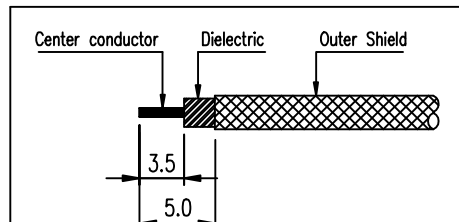
③번 CONNECTOR 단면도
