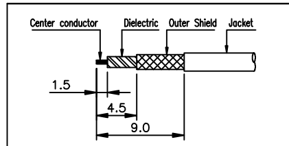
② CONNECTOR 단면도
