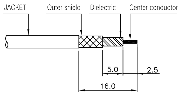
2번 Conn CABLE 탈피도
